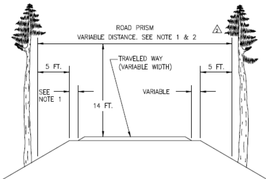
EXAMPLE 2 THRU FILL
